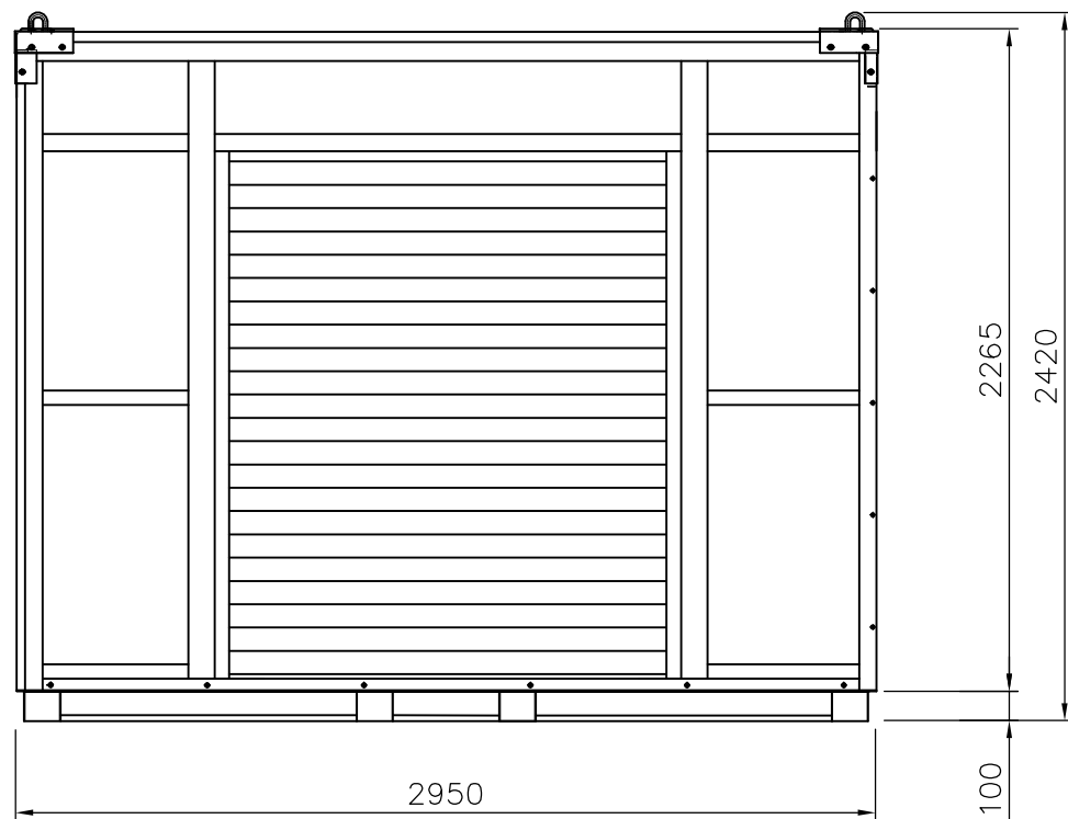
YO Elevation
